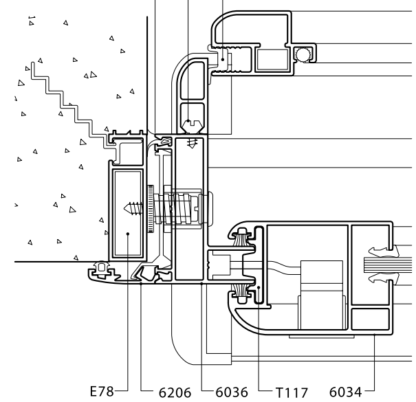
VC/PC Corte 1-2-3
