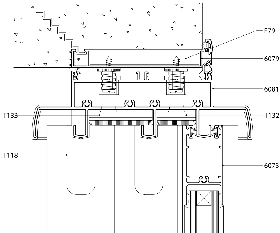
VC3/PC3 Corte 5
