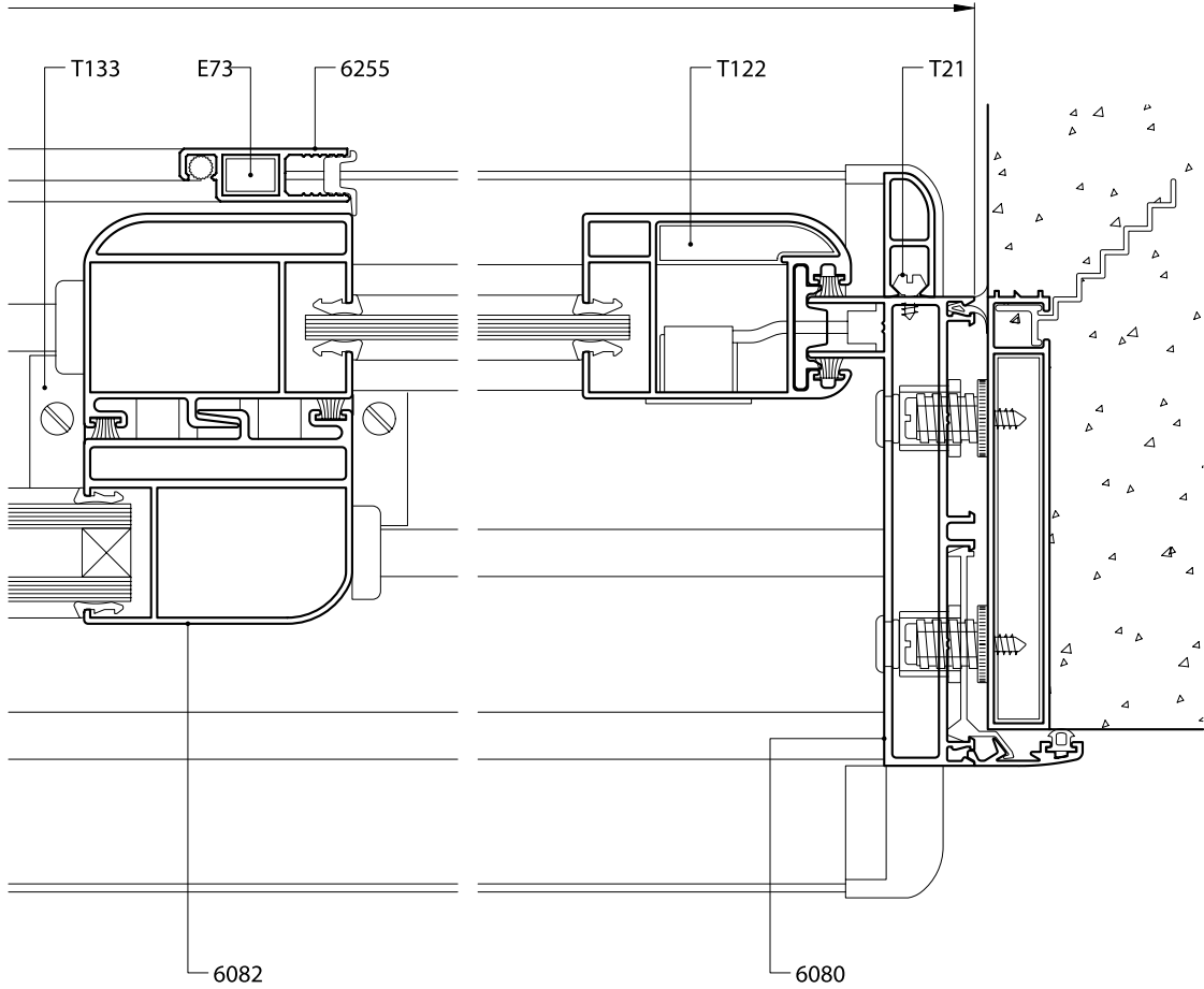
VC3 Corte 6
