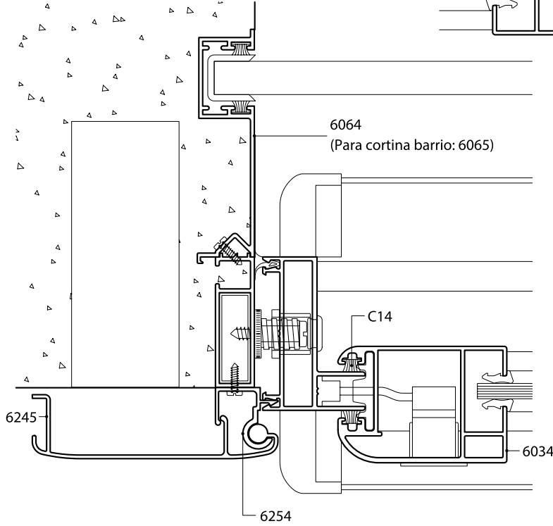
Detalle guía de cortina común
