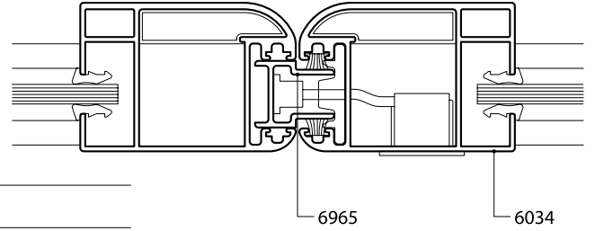
Detalle encuentro central 4 hojas
